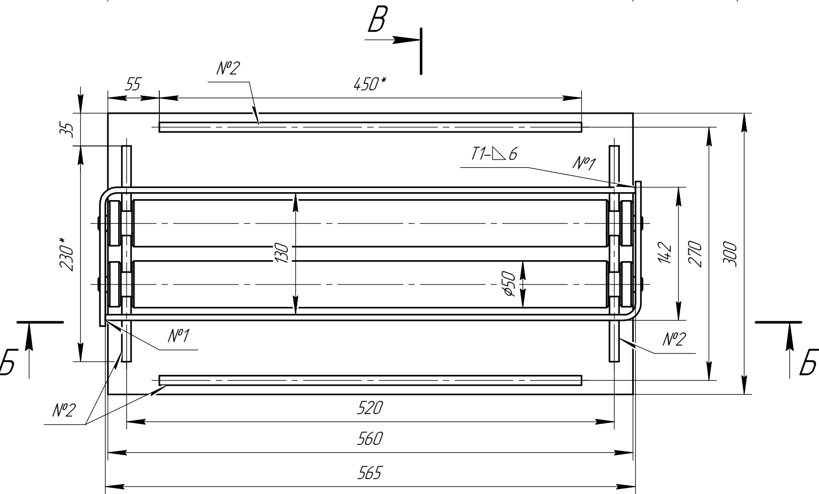
Det. poz. 1 (1:4)
