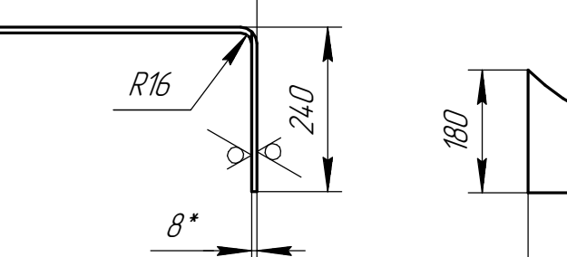
Det. poz. 2.3 (1:10)
