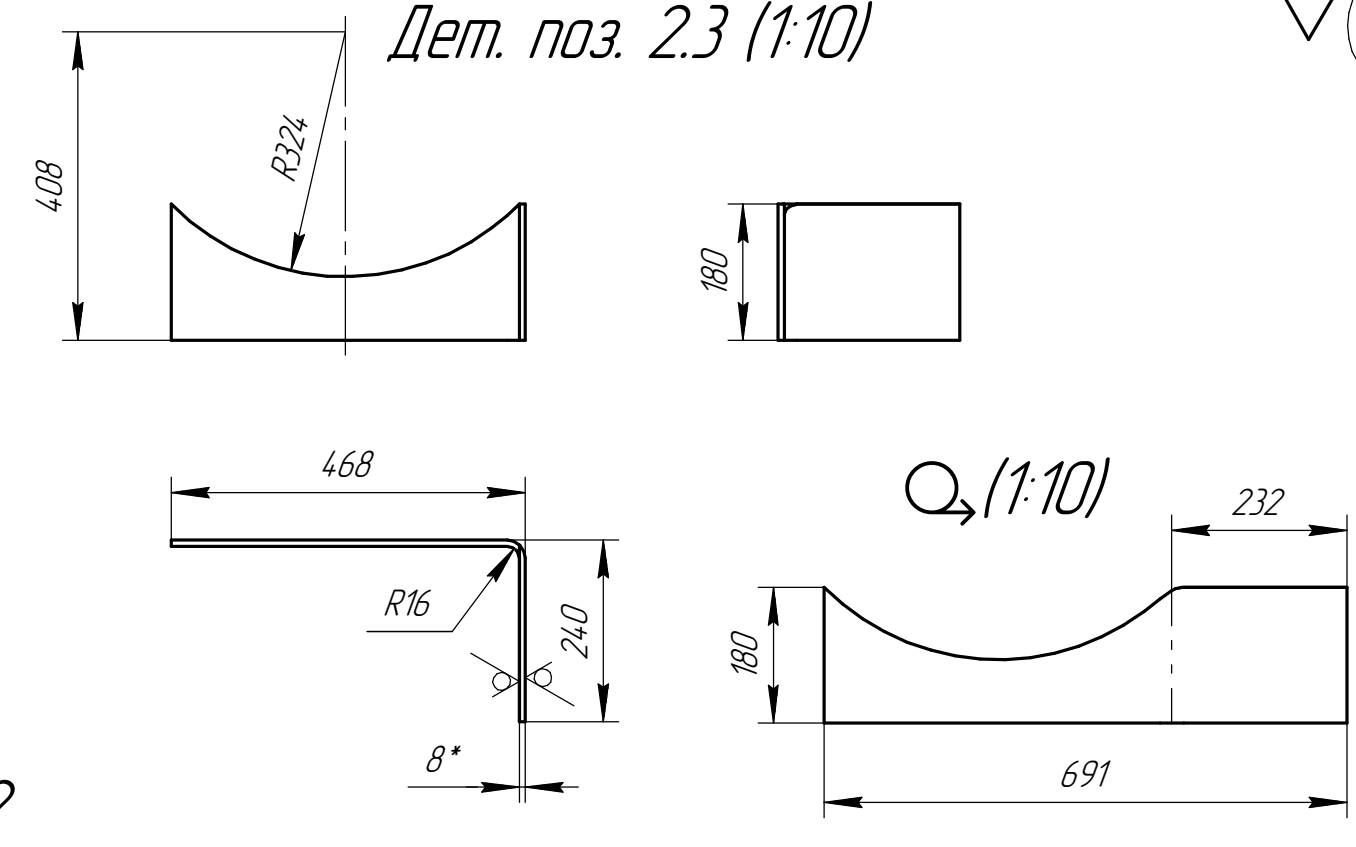
Det. poz. 2.3 (1:10)
