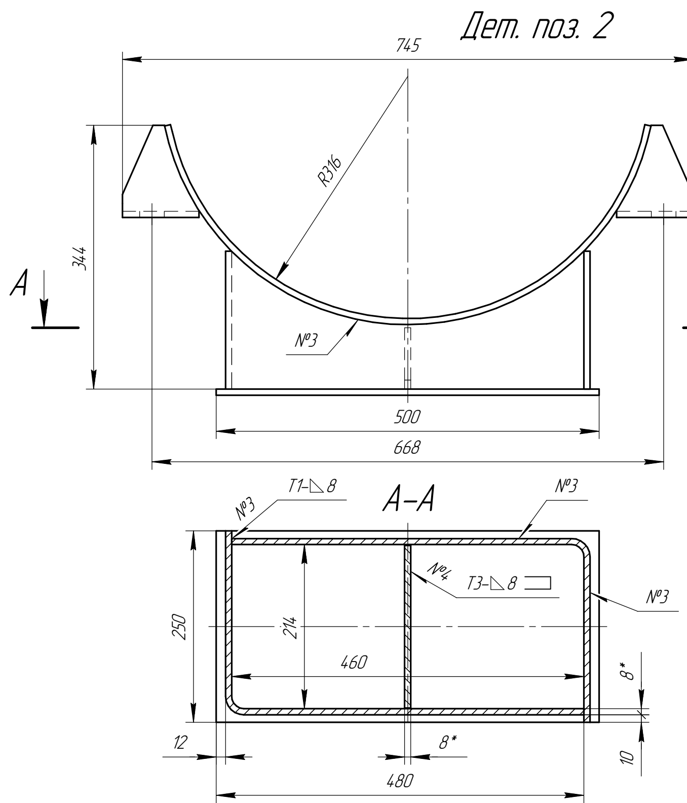
Det. poz. 2
