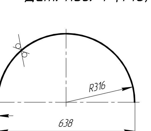
Det. poz. 1 (1:4)
