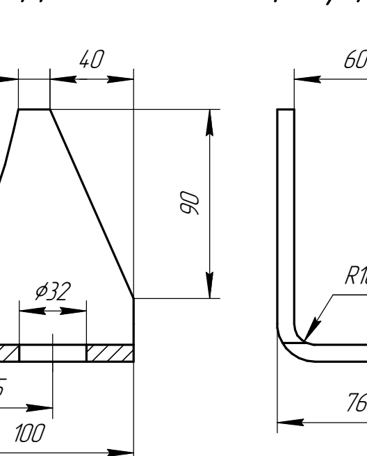
Det. poz. 2.4 (1:2,5)
