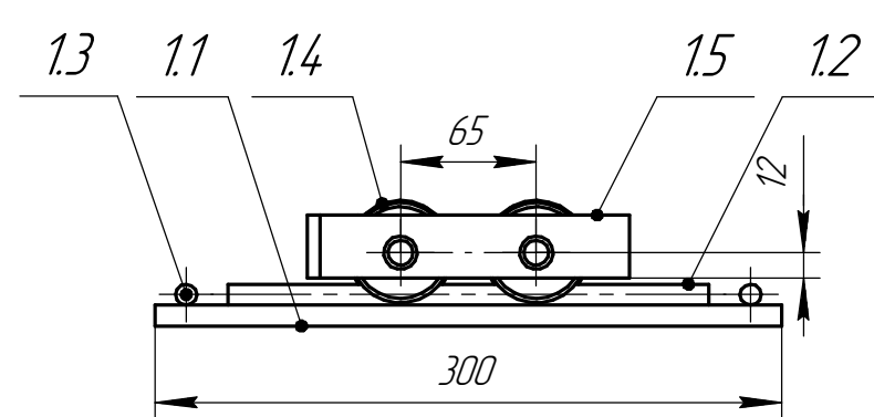
Det. poz. 1 (1:4)
