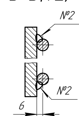
Det. poz. 1 (1:4)
